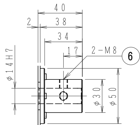
A部詳細
