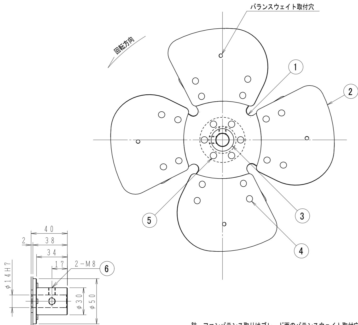
A部詳細
