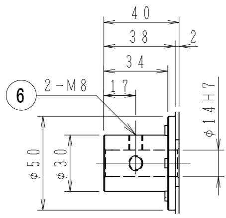
A部詳細
