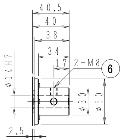
A部詳細
