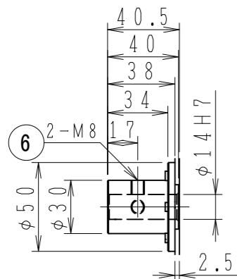
A部詳細
