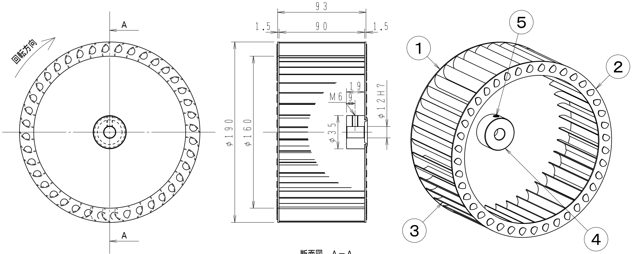
断面図 A-A
