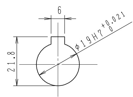
ボス穴詳細 (1:1)
