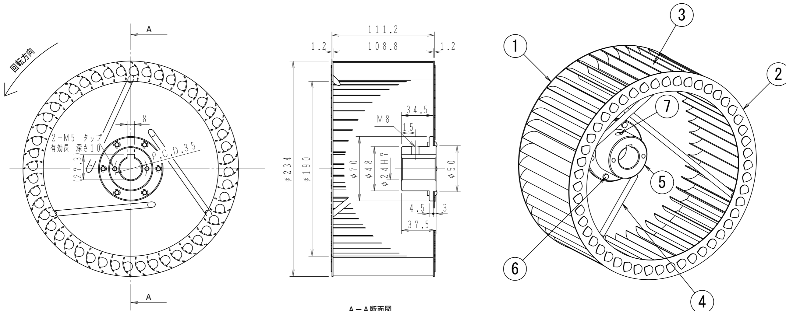
A-A断面図
