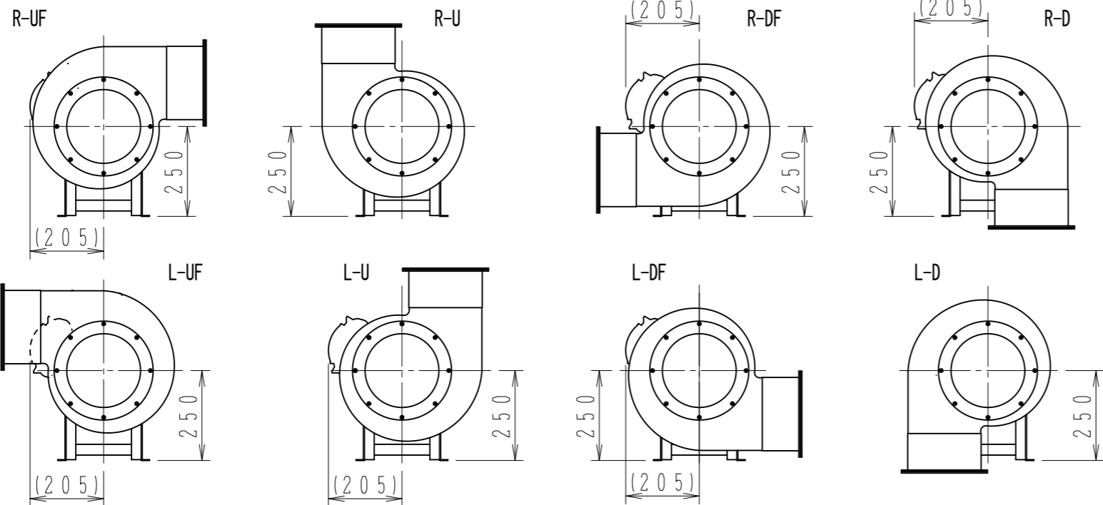
吐出方向一覧 (参考図) 主要寸法は上図と同じになります。
