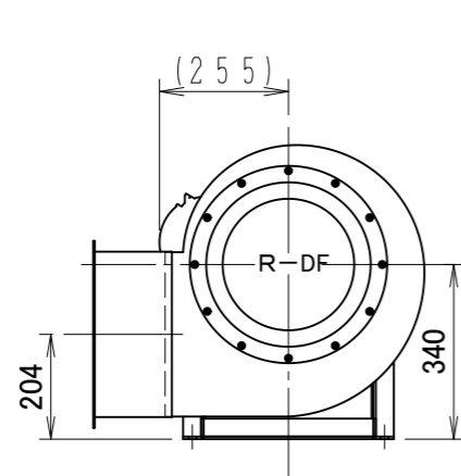
吐出方向一覧 (参考図)
