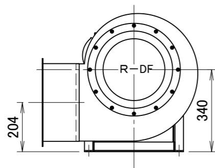
吐出方向一覧 (参考図)
